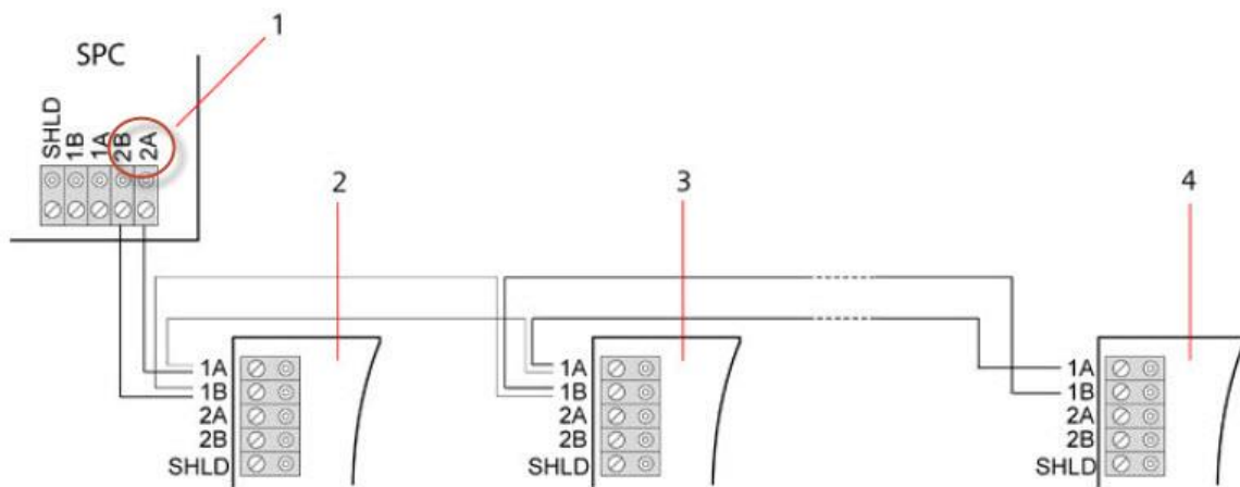
Multidrop-Konfiguration 2
