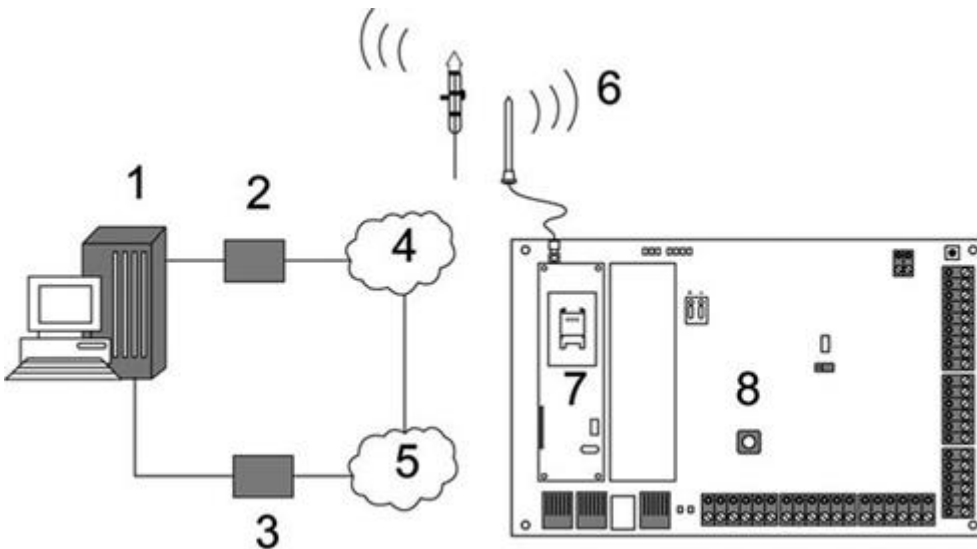
GSM-Verbindung
